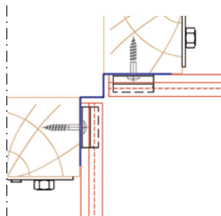
ANGLE RENTRANT AVEC PROFILÉ D'ANGLE
