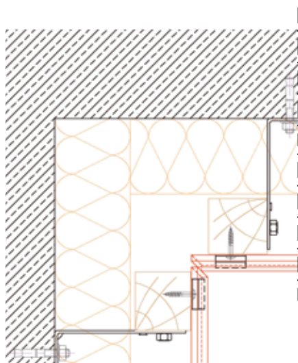
ANGLE RENTRANT
