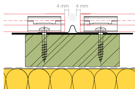
PROFIL DE JONCTION ABOUTAGE DES CLINS
