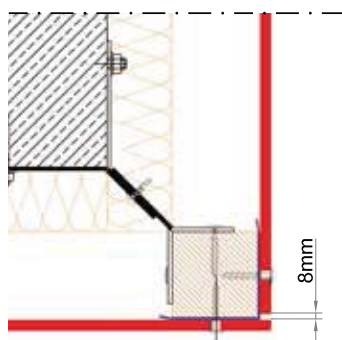
ANGLE SORTANT
