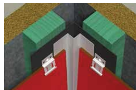
PROFIL D'ANGLE SORTANT CARRÉ
