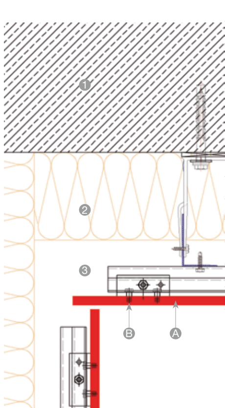
ANGLE RENTRANT
