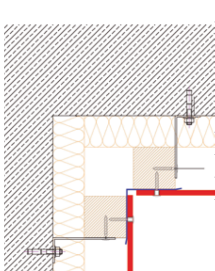
ANGLE RENTRANT
