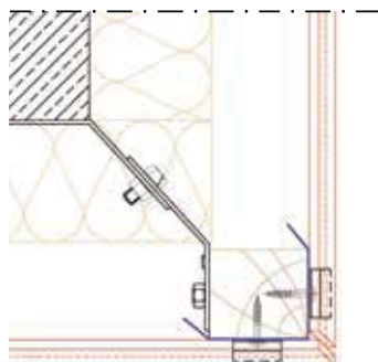
ANGLE SORTANT SANS PROFILÉ
