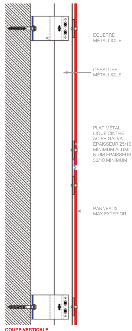
COUPE VERTICALE
