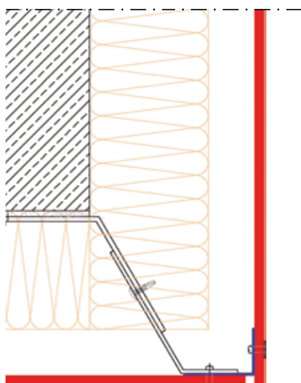
ANGLE SORTANT
