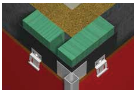
PROFIL D'ANGLE RENTRANT
