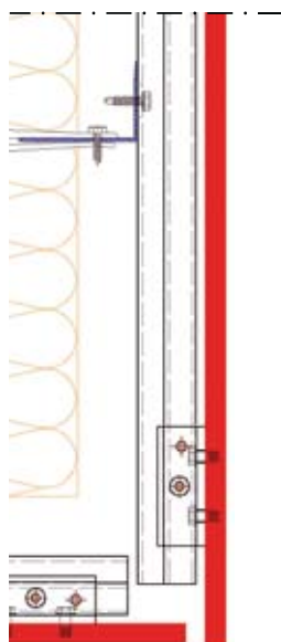
ANGLE SORTANT
