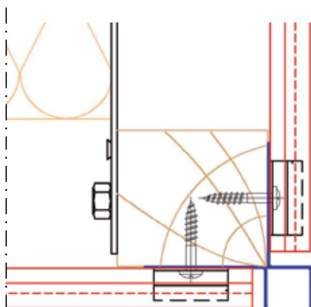
ANGLE SORTANT AVEC PROFILÉ CARRÉ
