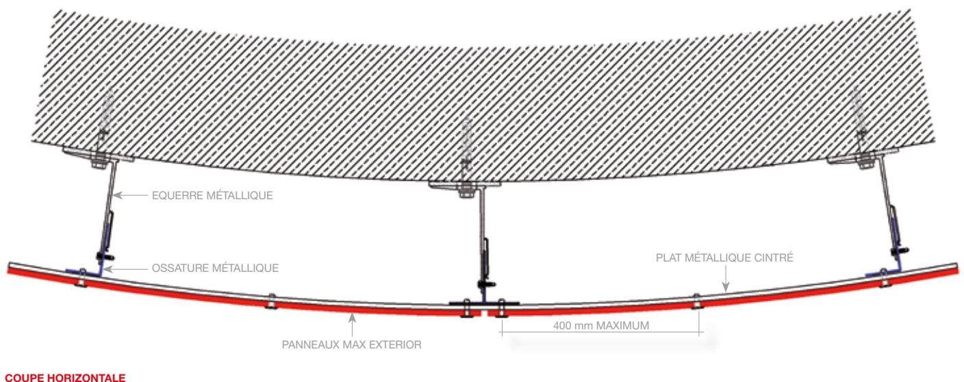
COUPE HORIZONTALE
