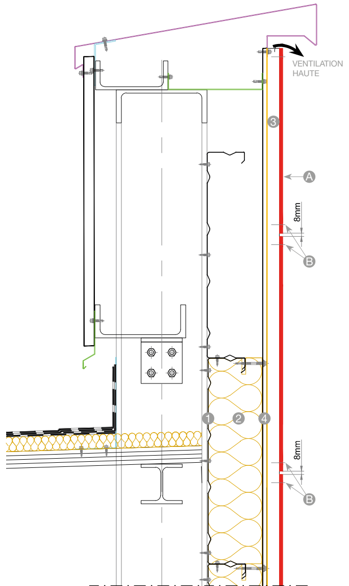
DÉTAILS POINT HAUT
