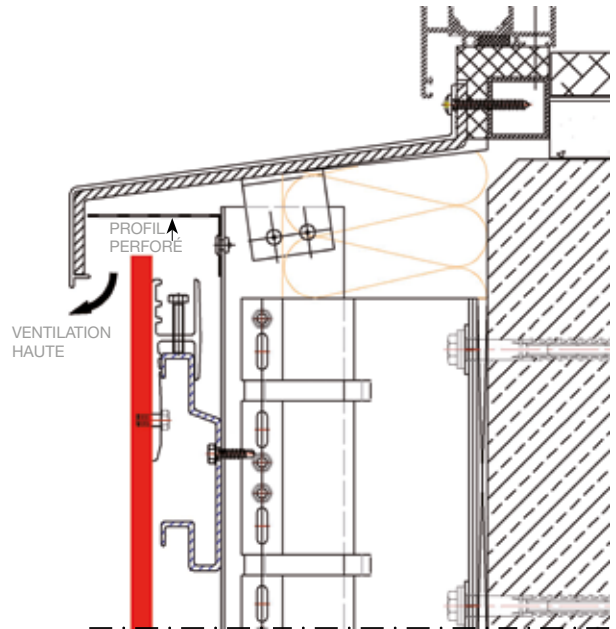
DÉTAIL APPUI DE FENÊTRE
