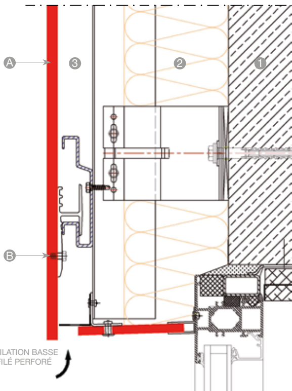
DÉTAIL LINTEAU
