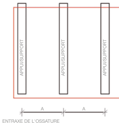
ENTRAIXE DE L'OSSATURE
