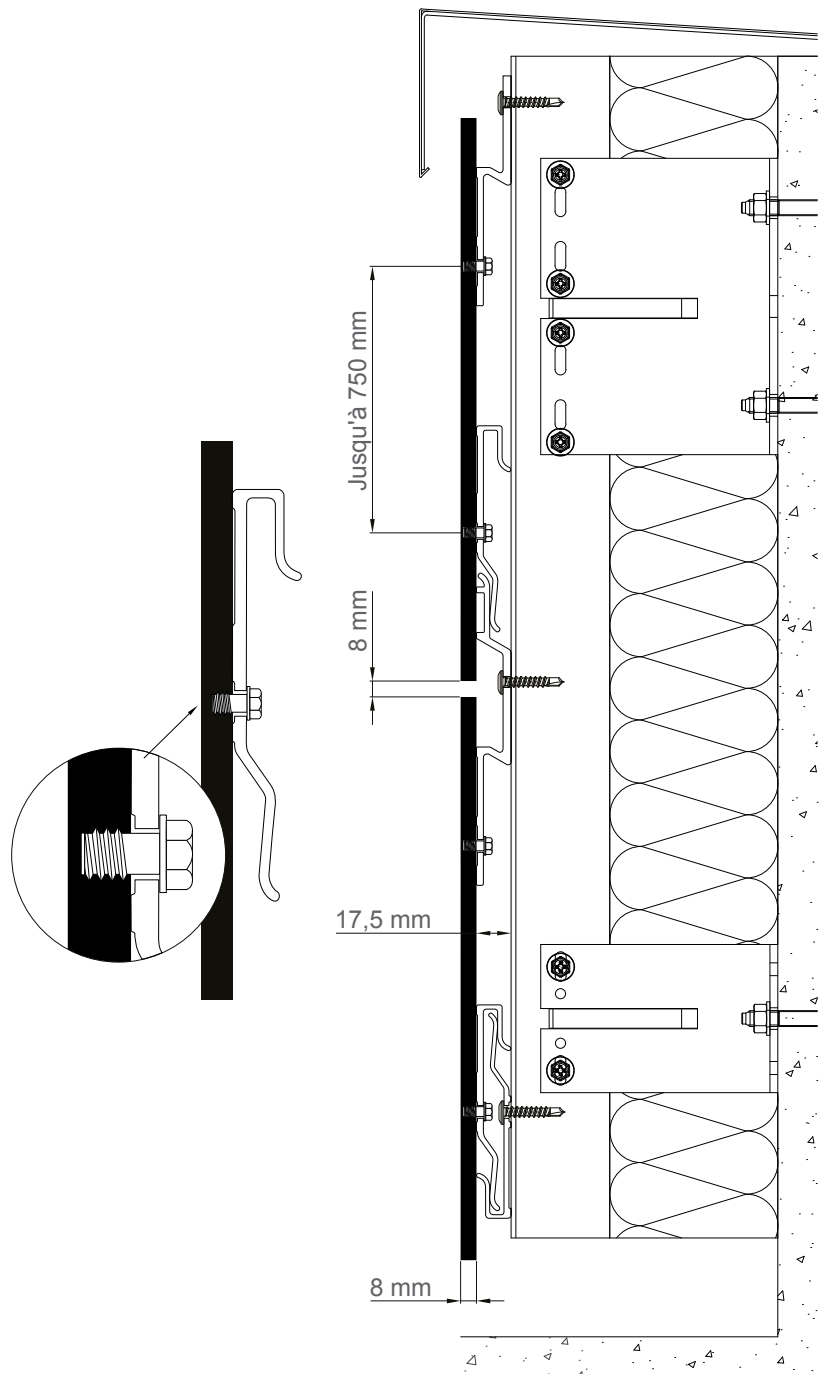
Montage avec Insert SFS Intec TU-S-6,0xL
